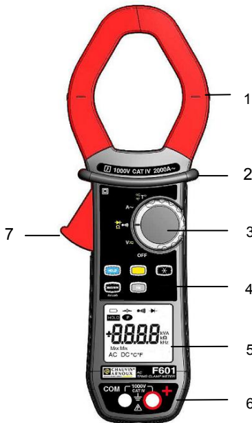
Abbildung 1 : Vielfachmesszange F601
